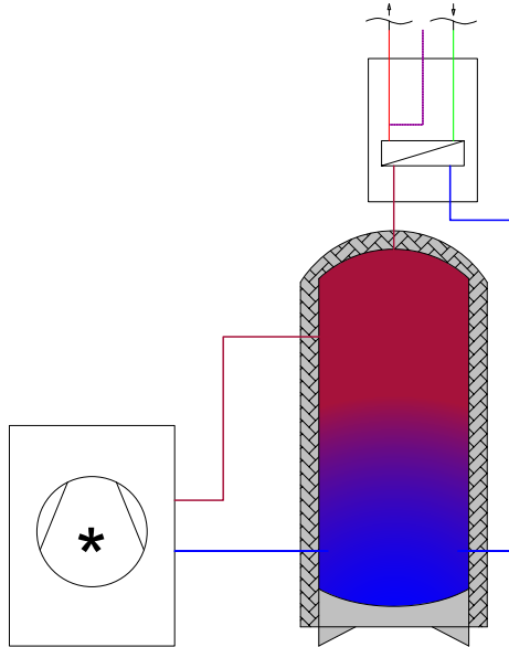
Abb. 1.12: Frischwasserstation
