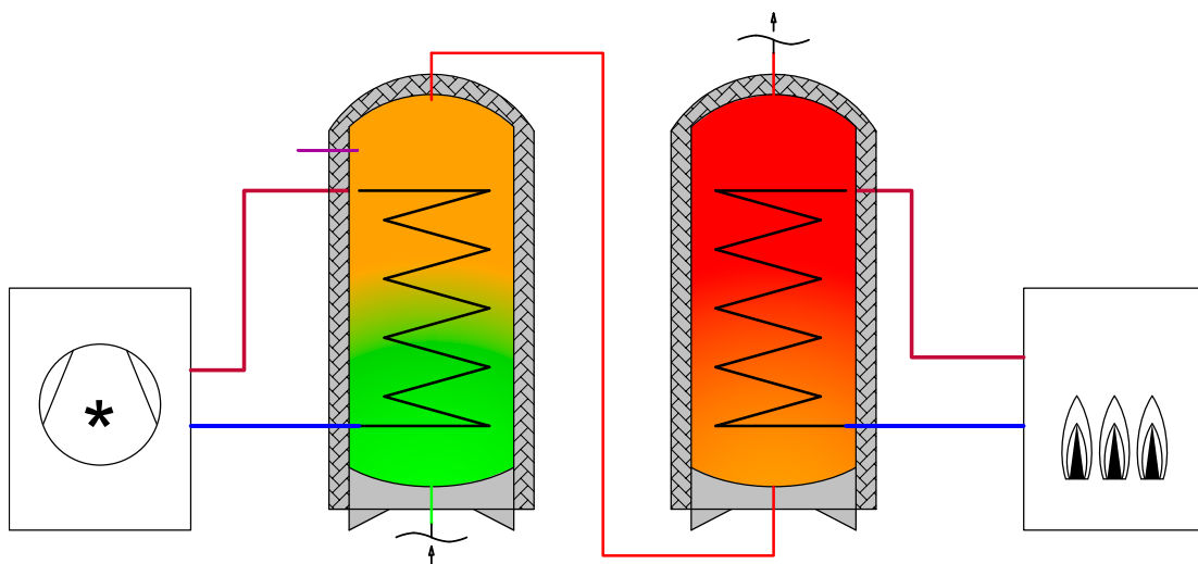
Abb.1.11: Bivalentes System mit Vorwärmstufe
