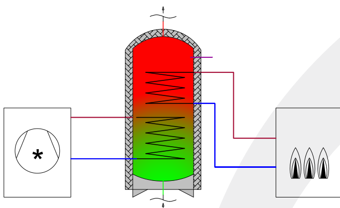
Abb.1.9.: Bivalenter Trinkwarmwasserspeicher mit zweitem Wärmeerzeuger
