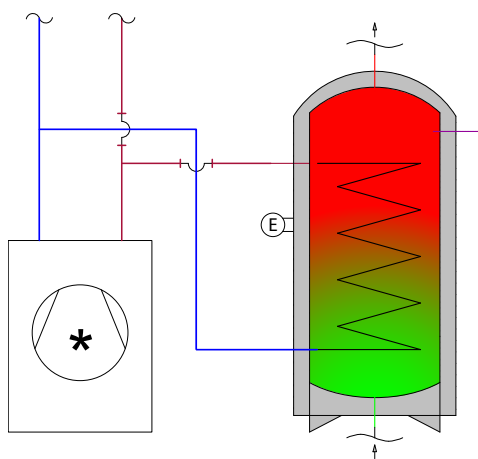
Abb.1.5.1: „Standard“-Wärmepumpe und Trinkwarmwasserspeicher mit integriertem Elektro-Heizstab
