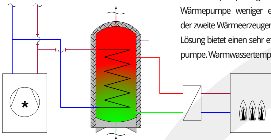
Abb.1.6: Trinkwarmwasserspeicher mit zweitem Wärmeerzeuger und externem Wärmeübertrager
