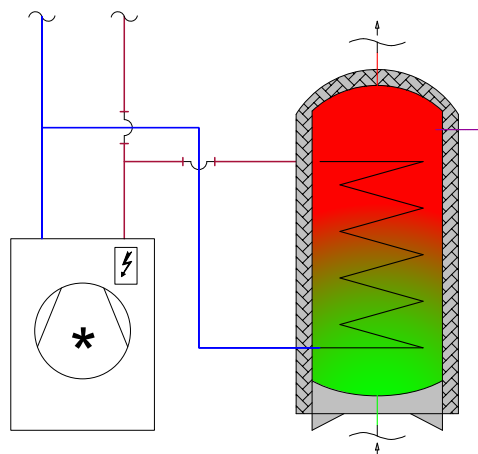
Abb.1.5.2: „Standard“-Wärmepumpe mit integriertem Elektro-Heizstab und Trinkwarmwasserspeicher
