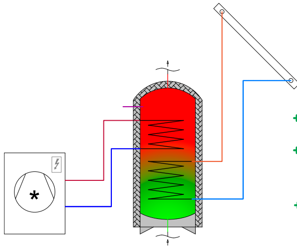
Abb.1.8.2: Bivalenter Trinkwarmwasserspeicher mit solarthermischer Anlage und Elektro-Heizstab in der Wärmepumpe
